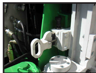
Verrouillage mât
